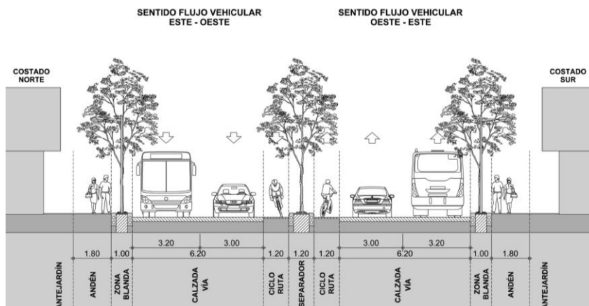
PERFIL TIPO KRA 1 D ENTRE CL 52 Y CL 56
