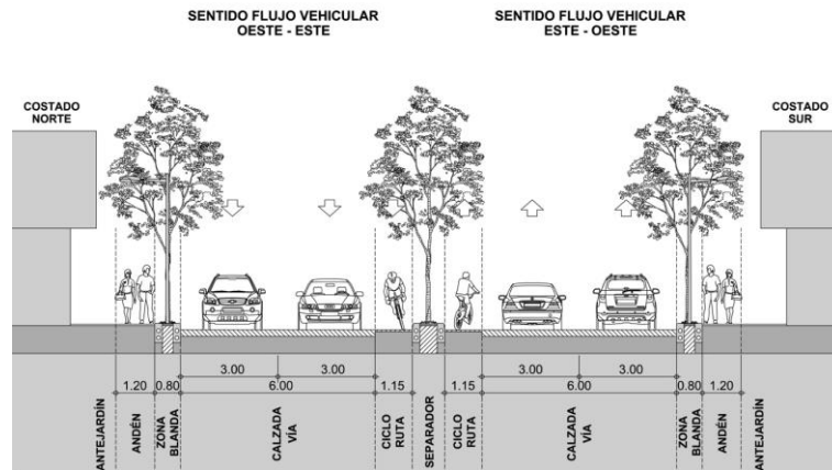
PERFIL TIPO CL 44 ENTRE KRA 1 Y KRA 5
