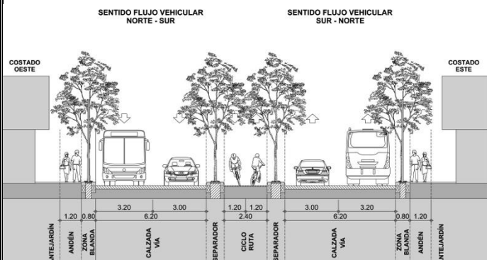
PERFIL TIPO CL 52 ENTRE KRA 6N Y KRA 1
