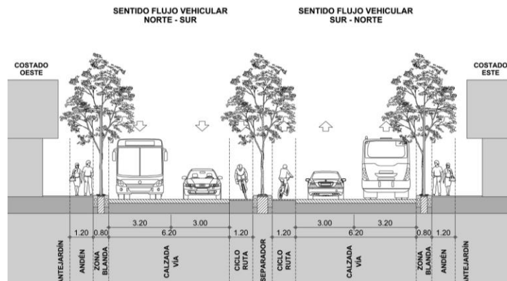
PERFIL TIPO CL 44 ENTRE KRA 1 Y KRA 5
